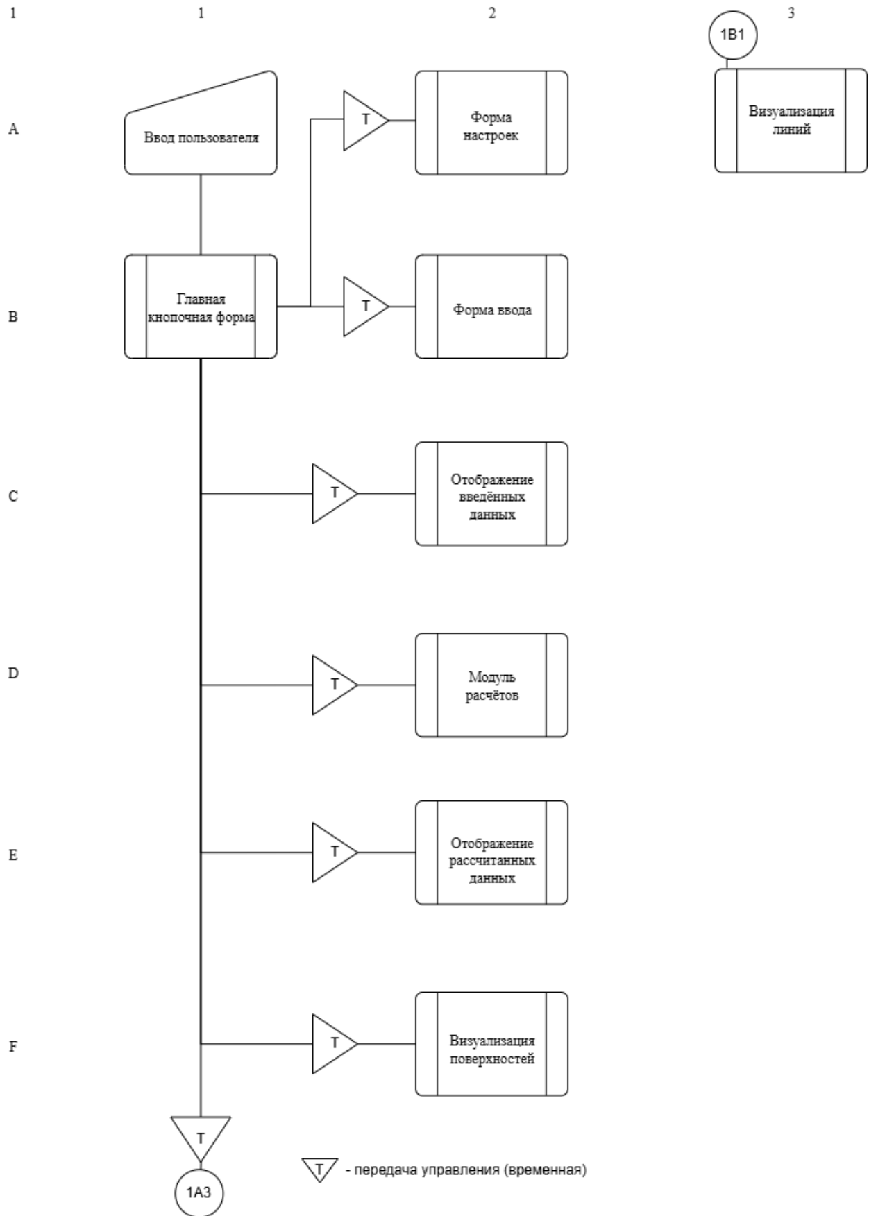
Рисунок 3.1. Схема взаимодействия программ
